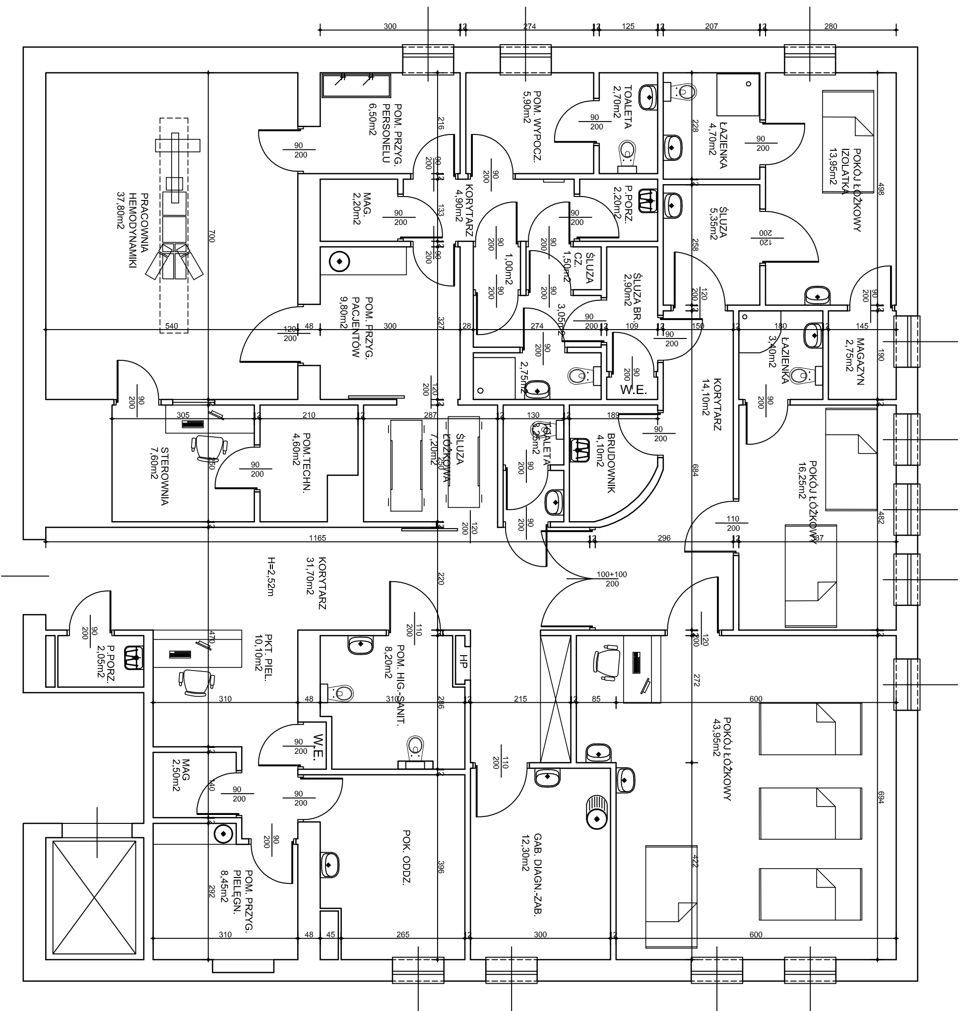
RYS. NR 2 FRAGMENT RZUTU DRUGIEGO PIĘTRA (ŚRODEK) STAN ISTNIEJĄCY
